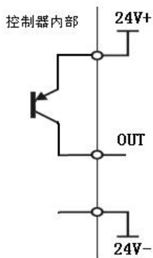
PNP型晶体管输出
