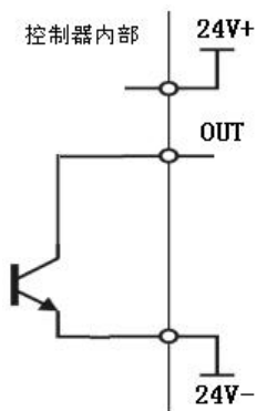
NPN型晶体管输出
