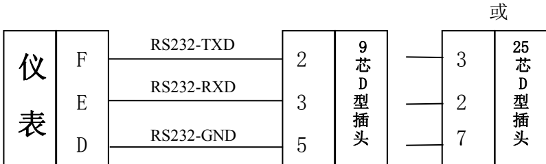
图 2.4 仪表与计算机连接示意图（RS-232 方式）
