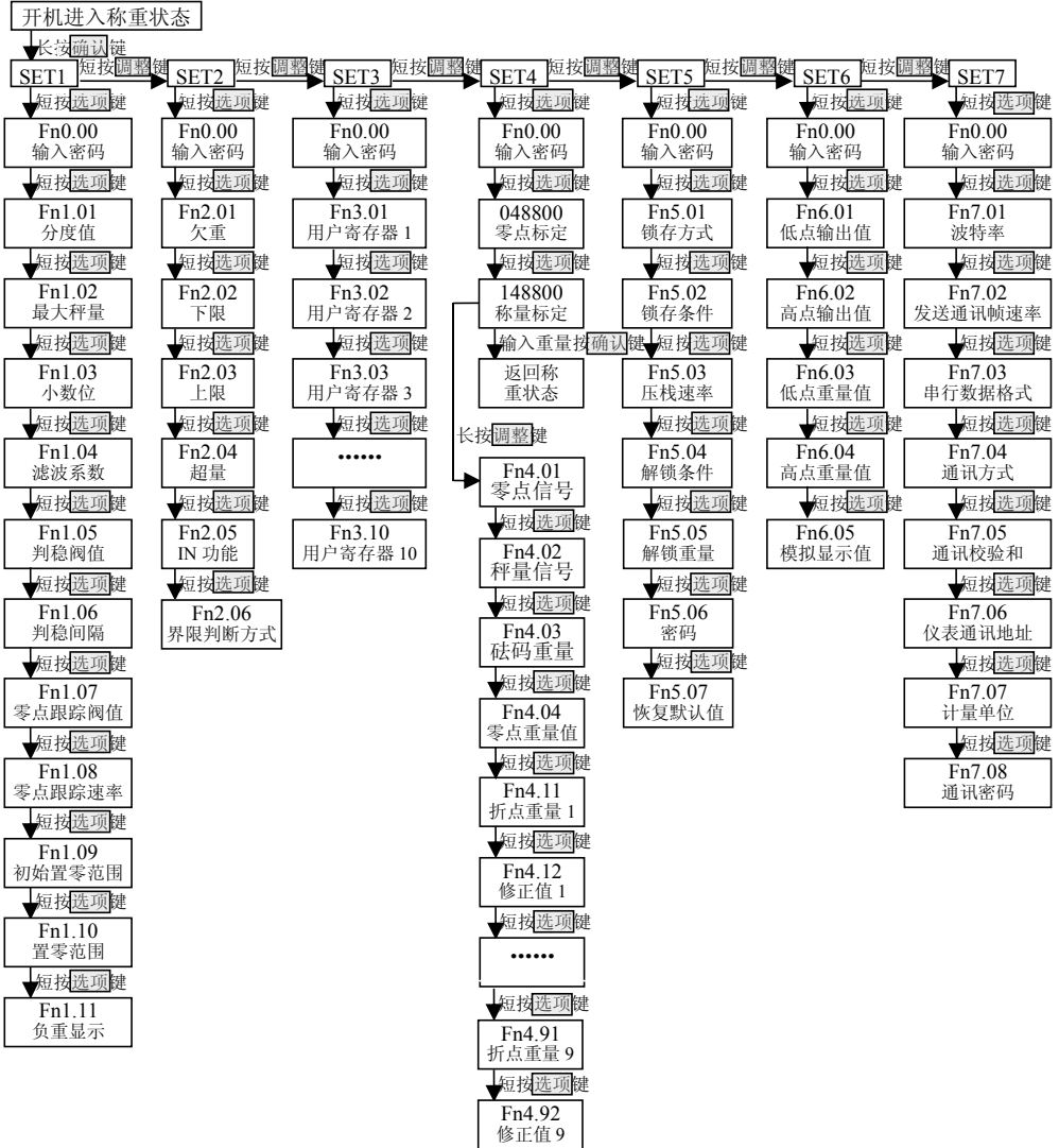
图 4.1 D13 各型仪表菜单结构
